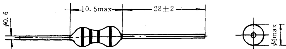
图 1 电感器的结构和外形尺寸
